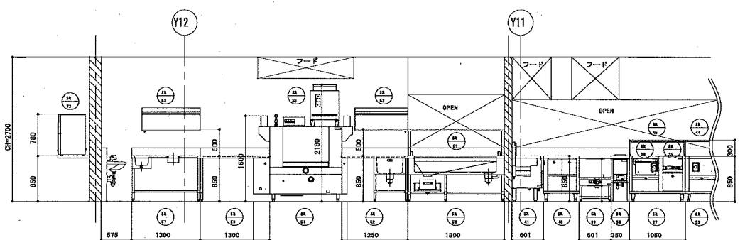
4-4断面
