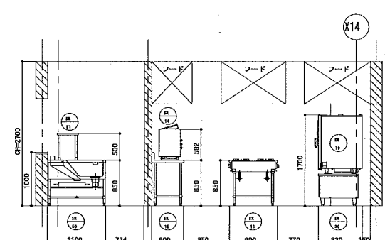
7-7断面
