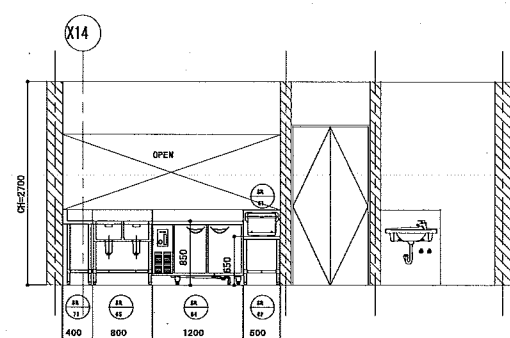
10-10断面
