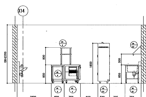
8-8断面
