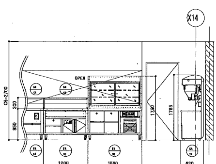
5-5断面
