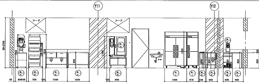
1-1断面
