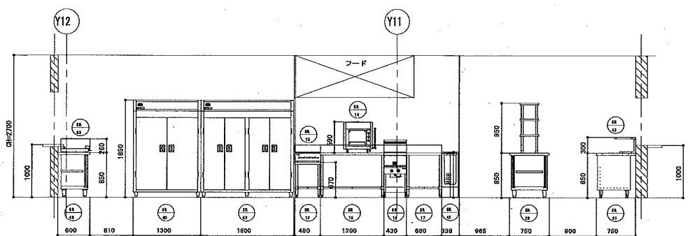
3-3断面
