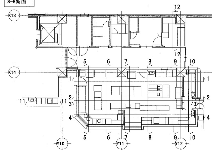
8-8断面
