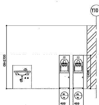
11-11断面
