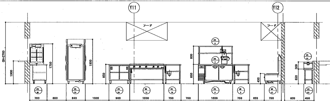
2-2断面
