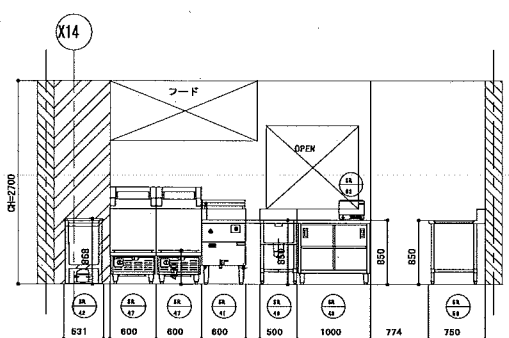
9-9断面
