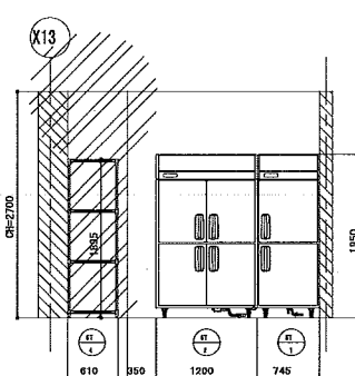
12-12断面
