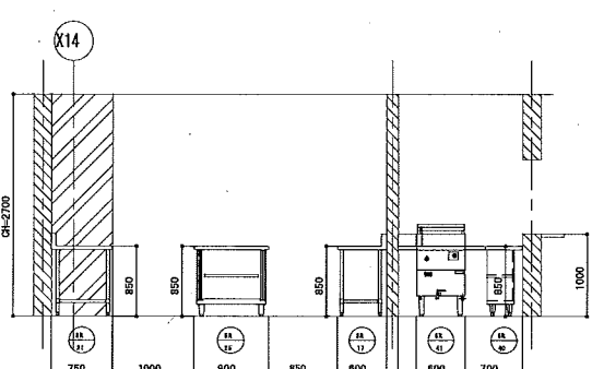
6-6断面
